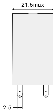
RKE2CO-LS正视图
