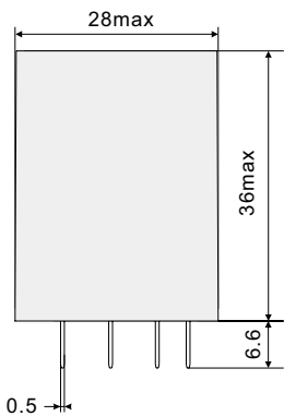
RKE2CO-LS/RKE4CO-LS侧视图
