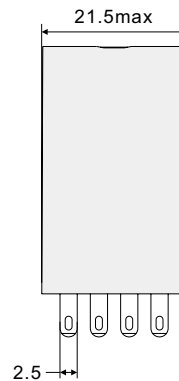
RKE4CO-LS正视图
